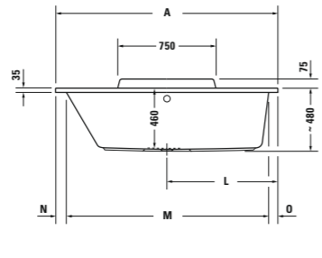
# 700292 00 0 00 0000, 1600 x 700 mm # 700294 00 0 00 0000, 1700 x 700 mm # 700296 00 0 00 0000, 1700 x 750 mm Einbauversion. Built-in. Da incasso. Version à encastrer. Inbouwversie. Versión empotrada *
